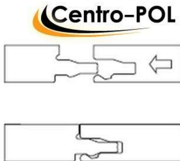
Рис.2. Lock-замок
