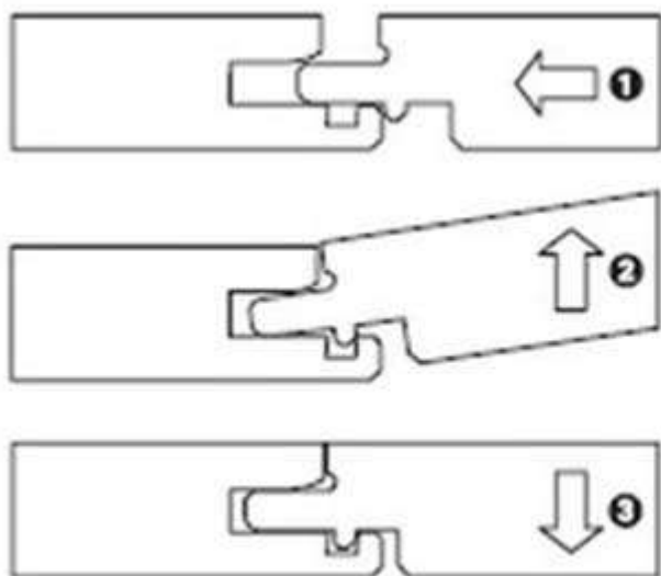
Рис.1. Click-замок
